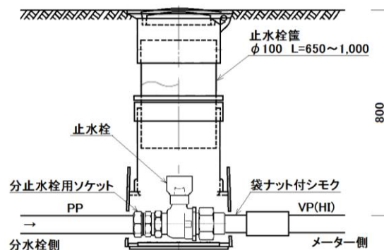
止水栓筐設置標準図(口径φ20～25mm)
