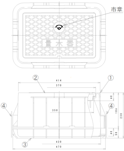
メーター口径 \phi 25\text{mm}
