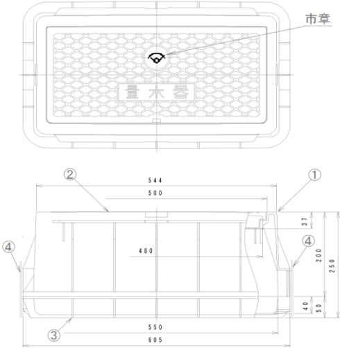
メーター口径 \phi 30\text{mm}
