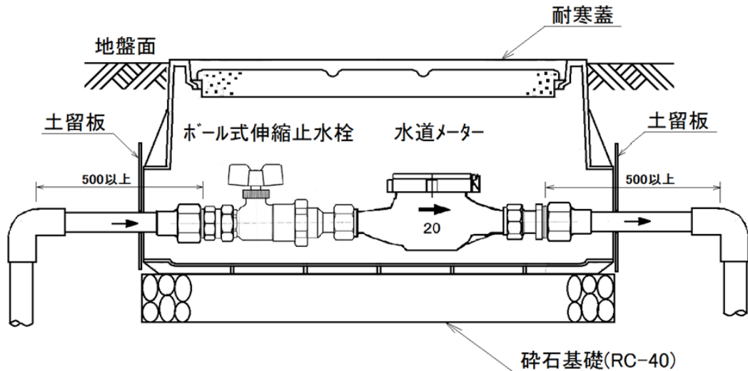
メーターボックス設置標準図 1 (メーター口径 \phi 13\sim 40\text{mm} 宅地内の場合)
