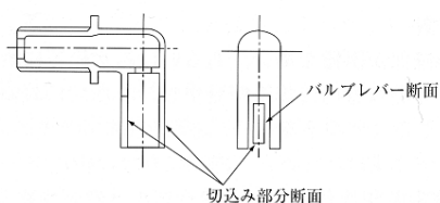
ボールタップの吐水口切り込み部分の断面
