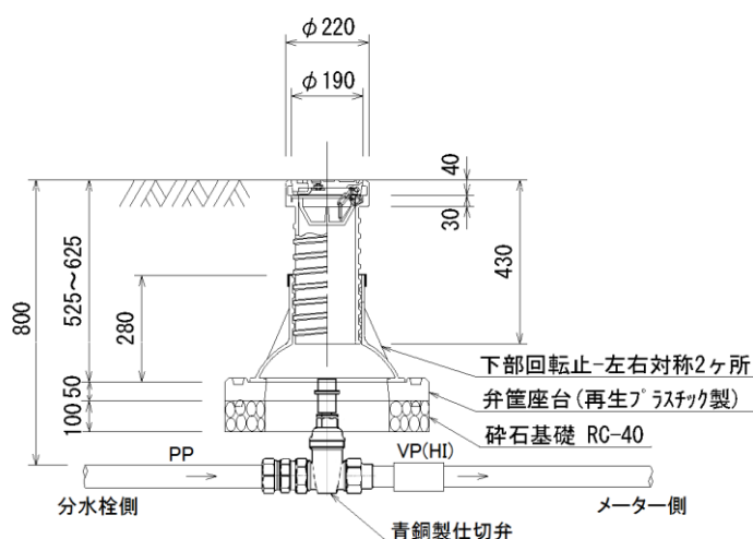
仕切弁
