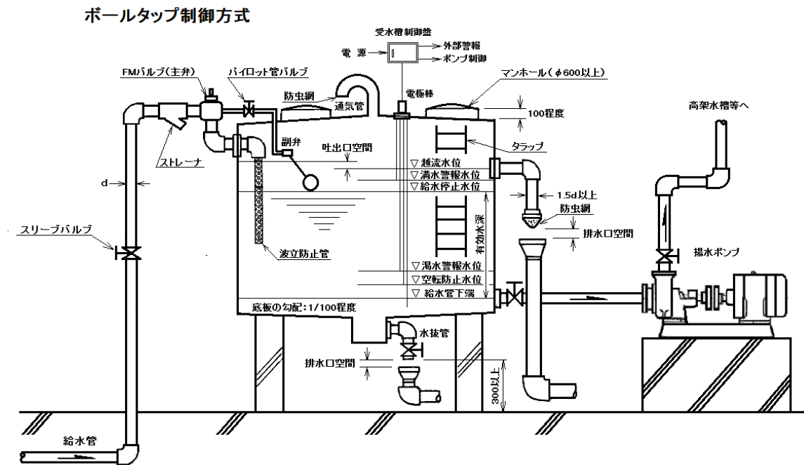
受水槽標準構造図
