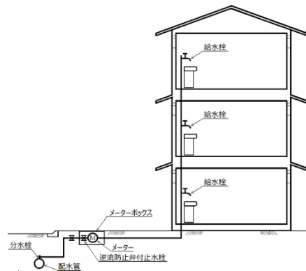
【直結直圧式(3 階)】
