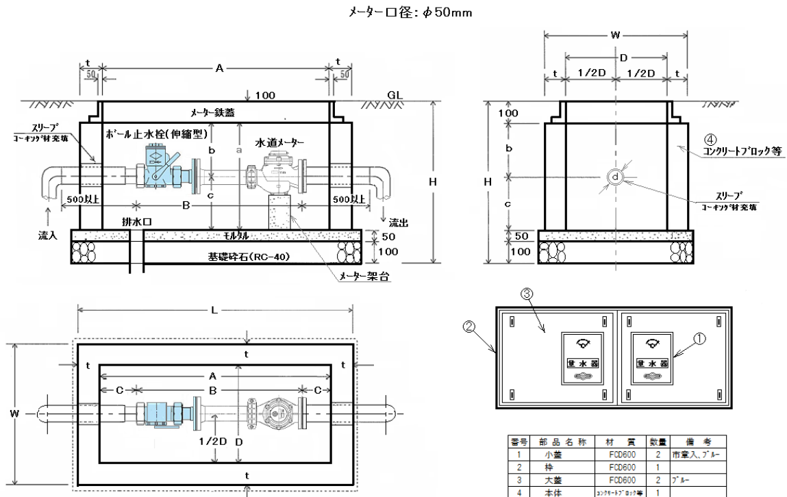
メーターボックス設置標準図3 (メーター口径φ50mm 以上歩道・私道の場合)
