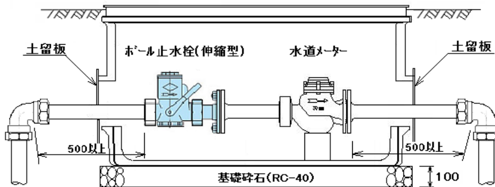
メーターボックス設置標準図2 (メーター口径φ50mm 宅地内の場合)
