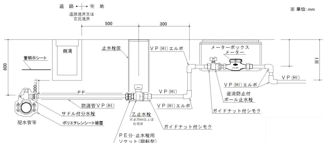
【サドル分水栓による分岐方法（配水管等埋設深800mmの場合）】
