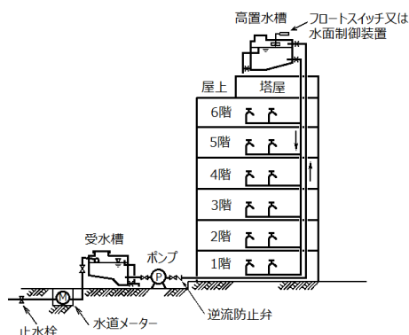
【高置水槽式】
