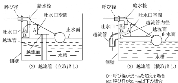
水槽等の場合
