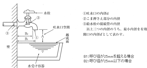
洗面器等の場合
